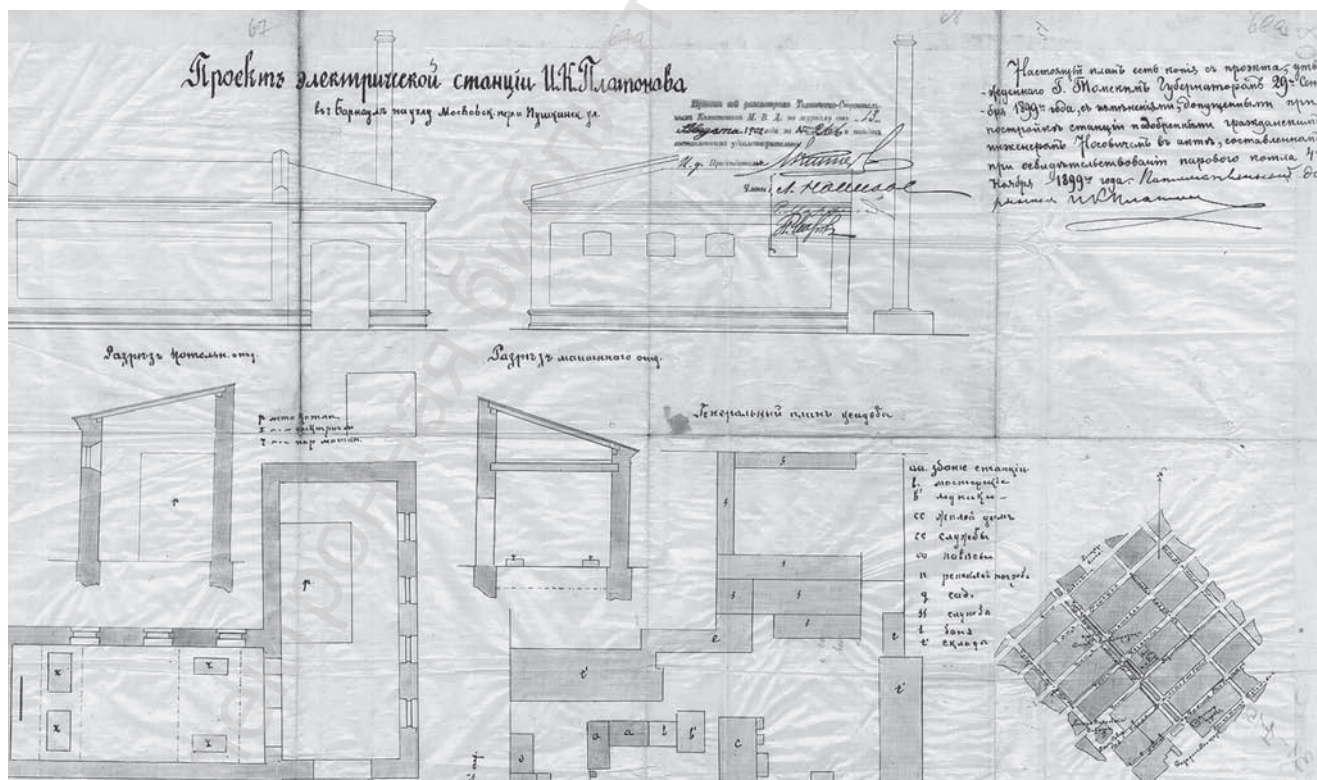
Проект электрической станции И. К. Платонова в г. Барнауле между Московским переулком и Пушкинской улицей с изменениями, допущенными при постройке станции и одобренными гражданским инженером И. Ф. Носовичем актом от 4 ноября 1899 г. ГААК. Ф. 31. Оп. 1. Д. 158. Л. 68. Рукописный подлинник.
