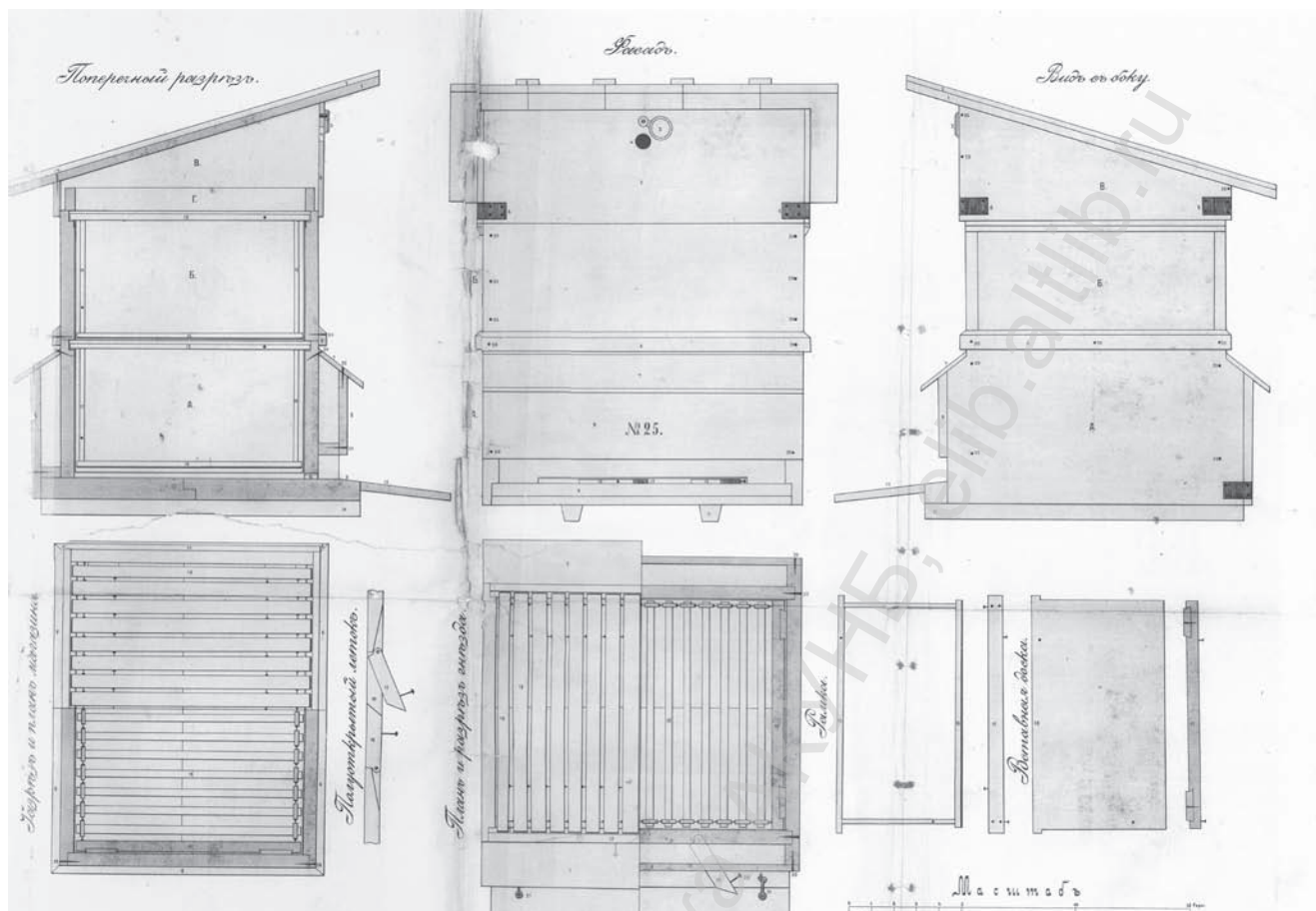
Конструкторский чертеж улья системы «Сибиряк», изготовленный в мастерской пчеловодных принадлежностей Алтайского округа. 1900 г. ГААК. Ф. 4. Оп. 1. Д. 180. Л. 164. Подлинник.
