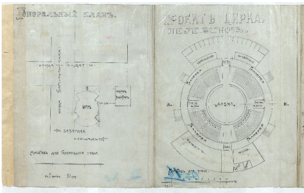
Проект цирка А.Г. Коромыслова. 1914. ГАНО. Ф. Д-97. Оп.1. Д.57.
