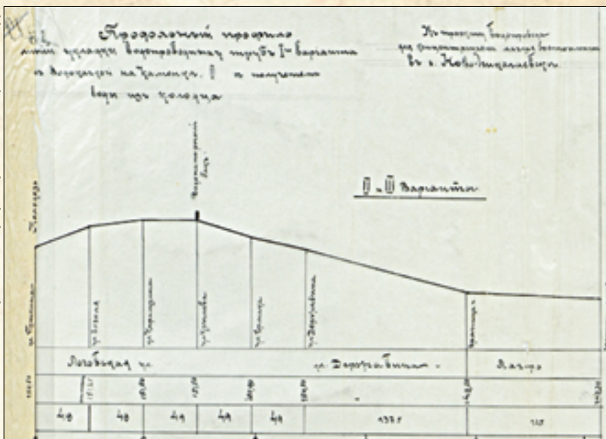
Илл. 4. Продольный профиль укладки водопроводных труб
