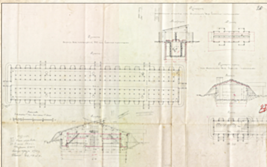
Илл. 3. Проект барака, отхожего места и кухни концлагеря
