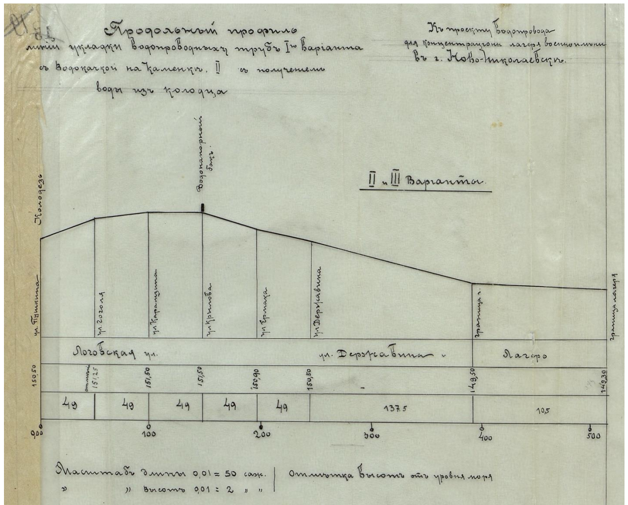
Илл. 4. Продольный профиль укладки водопроводных труб 13
